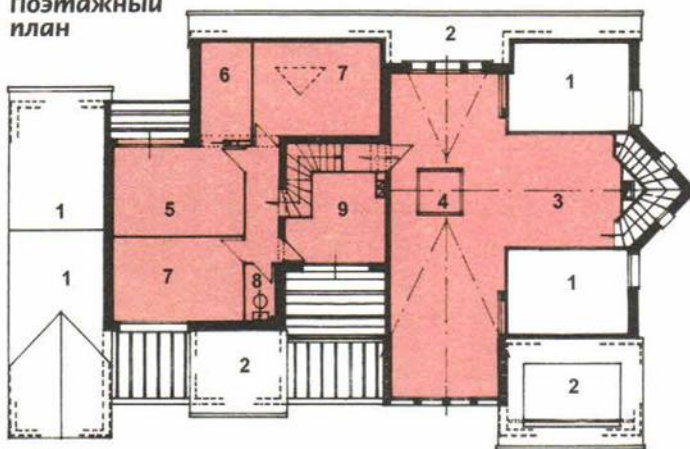
Планировка помещений 1-го этажа:
